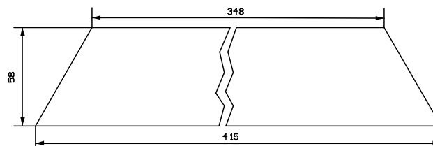
Fußteil D - Foot part D
