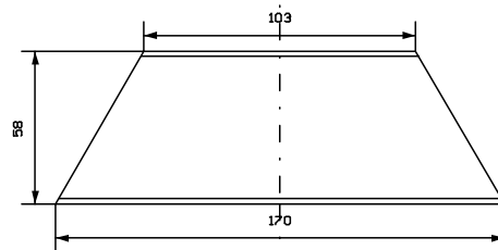
Fußteil C -Foot part C
