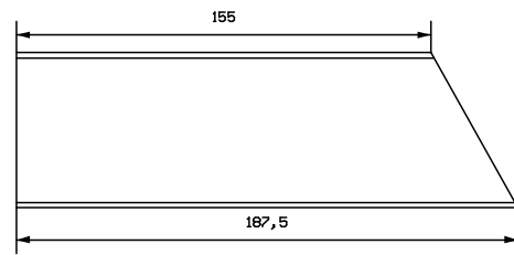
Fußteil B - Foot part B
