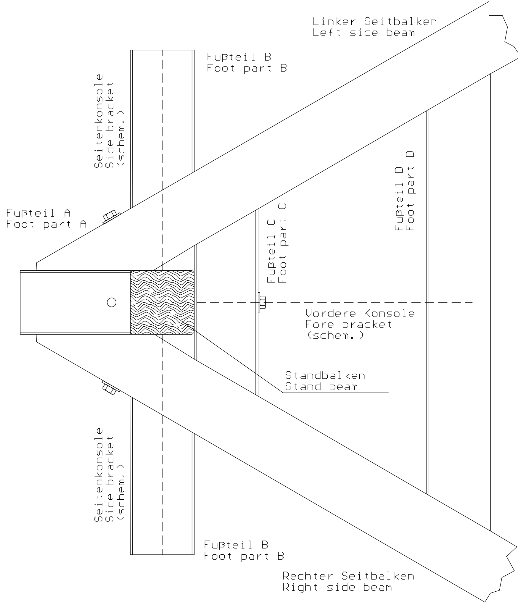
Standfuß - Draufsicht - Montagedarstellung
